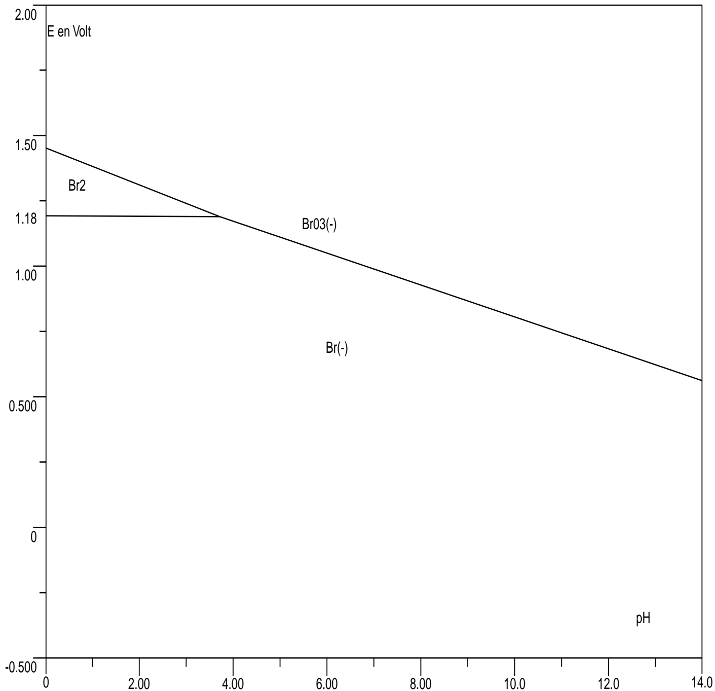
Diagramme simplifié potentiel-pH du brome
